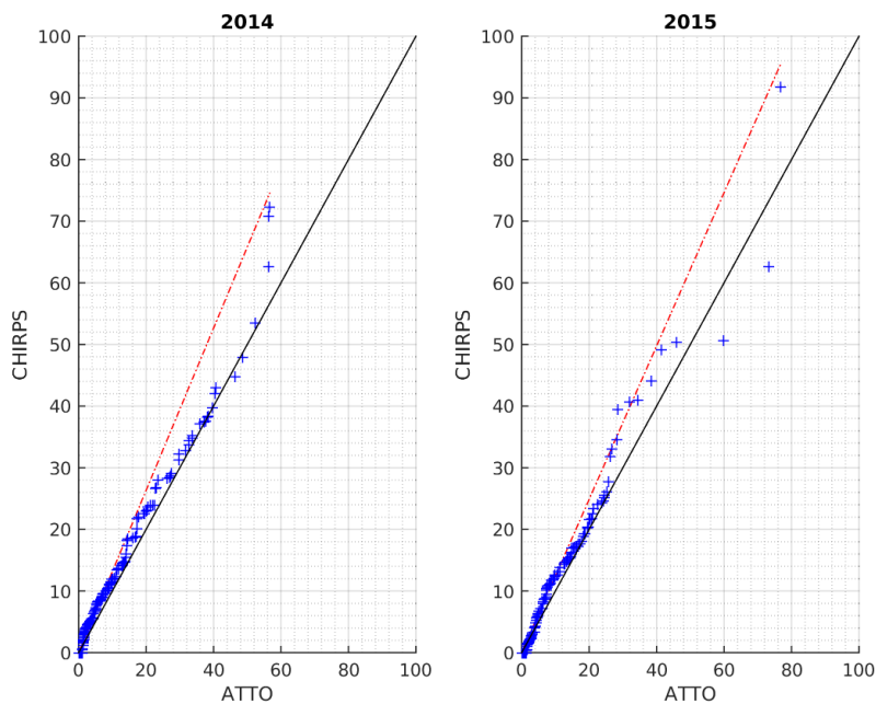
Figura 15: Q-q plots dos dados diários de precipitação do CHIRPS e da estação ATTO, para 2014 e 2015. A linha contínua preta representa a linha 1:1 e a tracejada vermelha o ajuste linear.
