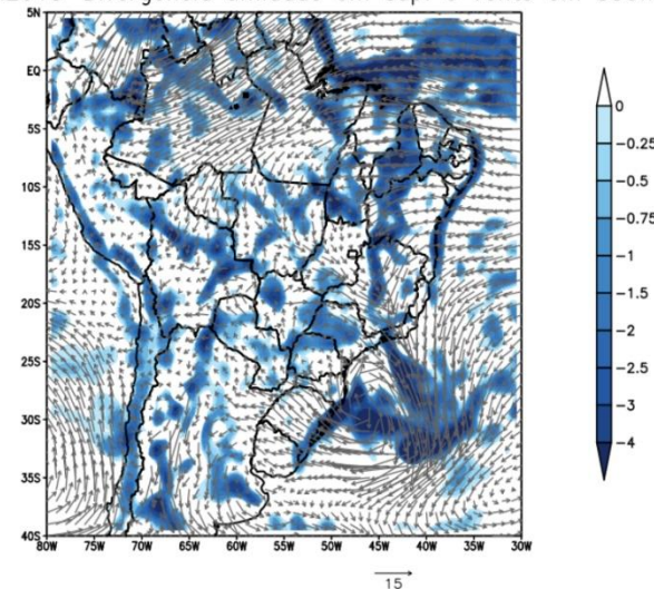
Figura 62: Campos sinóticos referentes ao dia 11/03/2015 as 06Z. (a) Linhas de corrente e divergência ( 10^{-5} \text{ s}^{-1} ) em 200hPa. (b) Ômega (Pa/s) e altura geopotencial (gpm) em 500 hPa. (c) Divergência de umidade ( 10^{-4} \text{ g/kg/s} ) em superfície e vento (m/s) em 850 hPa. (d) Temperatura ( ^{\circ}\text{C} ), PRNM (hPa) e vento (m/s) em 1000hPa. A ATTO está indicada com um quadrado preto, INMET com um círculo preto e o MAO com um triângulo preto nos mapas.
