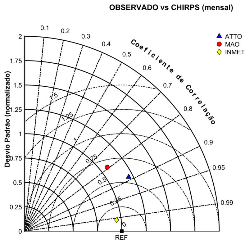
Figura 33: Diagrama de Taylor para as séries mensais de precipitação referentes às estações ATTO (triângulo azul), MAO (círculo vermelho) e INMET (losango amarelo). As variáveis foram todas normalizadas pelo desvio padrão das observações.
