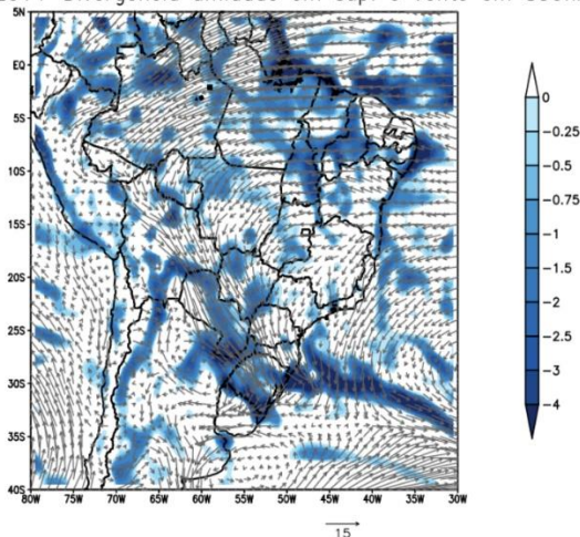
Figura 53: Campos sinóticos referentes ao dia 19/03/2014 as 12Z. (a) Linhas de corrente e divergência ( 10^{-5} \text{ s}^{-1} ) em 200hPa. (b) Ômega (Pa/s) e altura geopotencial (gpm) em 500 hPa. (c) Divergência de umidade ( 10^{-4} \text{ g/kg/s} ) em superfície e vento (m/s) em 850 hPa. (d) Temperatura ( ^{\circ}\text{C} ), PRNM (hPa) e vento (m/s) em 1000hPa. A ATTO está indicada com um quadrado preto, INMET com um círculo preto e o MAO com um triângulo preto nos mapas.
