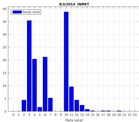
Figura 52: Variação horária da (a) precipitação; (b) umidade relativa; (c) temperatura do ar; (d) pressão; (e) velocidade do vento; e (f) direção do vento, para o dia 08/03/2014 da estação INMET.
